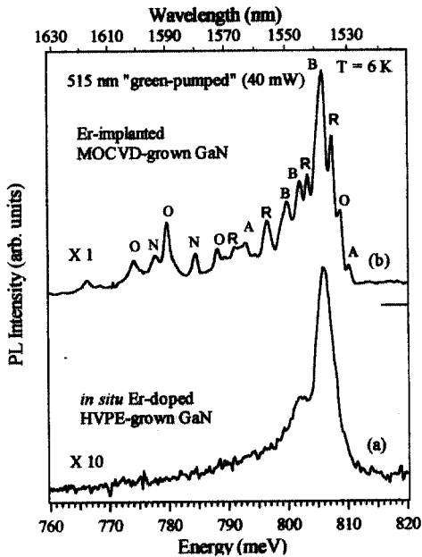
그림 1. 515nm로 펌핑시킨 Er^{3+} 의 {}^4I_{13/2} \rightarrow {}^4I_{11/2} 발광에 대한 PL 스펙트럼 (a) In situ Er 도핑된 GaN (b) Er이 이온주입된 GaN. Fig. 1. {}^4I_{13/2} \rightarrow {}^4I_{11/2} emissions of Er^{3+} in the PL spectra pumped by 515nm wavelength light (a) In situ Er doped GaN (b) Er-implanted GaN.
