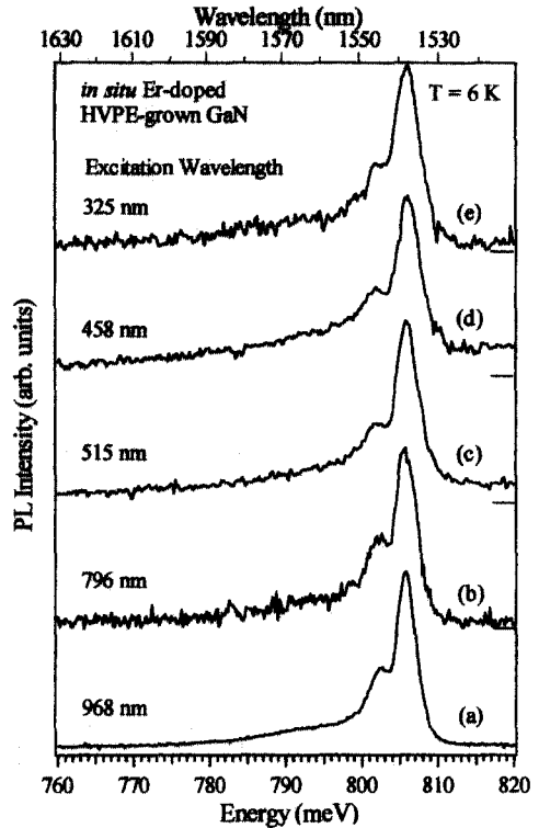
그림 8. 여러 파장으로 여기시킨 in situ Er 도핑된 GaN의 PL 스펙트럼의 비교.
