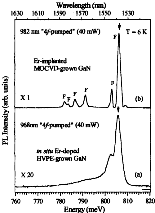
그림 7. 4f-band로 직접 여기시킨 PL 스펙트럼 (a) 968nm의 파장으로 여기시킨 in situ Er 도핑된 GaN의 PL 스펙트럼 (b) 982nm의 파장으로 여기시킨 Er이 이온주입된 GaN의 PL 스펙트럼.
