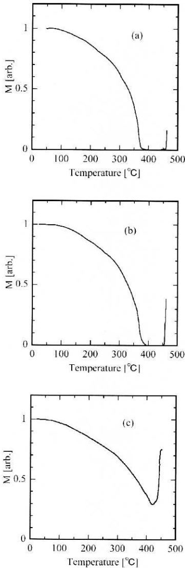
그림 1. (\text{Fe}_{1-x}\text{Co}_x)\text{76Si}_{11}\text{B}_{13} 아몰퍼스 박막에 있어서 자화의 온도 의존성; (a) x = 0 , (b) x = 10 , (c) x = 20 .
