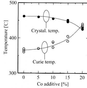
그림 2. \text{FeCoSiB} 박막에서의 Co 함량에 따른 큐리온도와 결정화온도의 변화.
