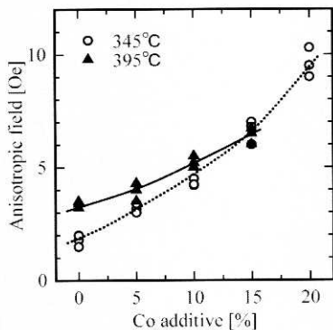
그림 3. FeCoSiB 박막에서의, Co 함량에 따른 이방성자계의 변화.
