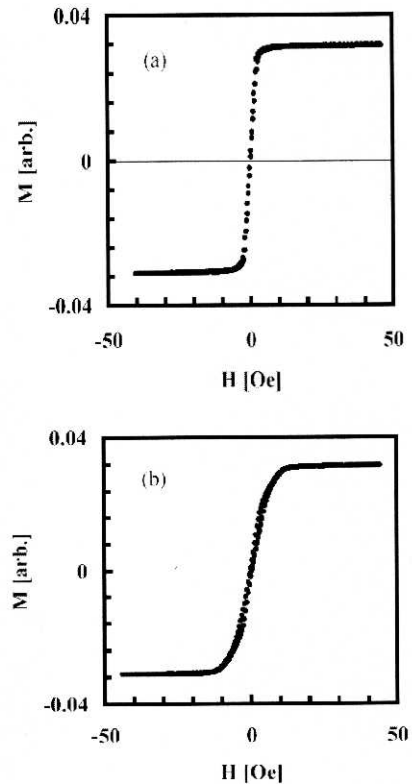
그림 4. 395 ° C에서 열처리된 FeCoSiB 박막(Co 함량 10 %)의 자화곡선; (a)는 자화용이축방향으로, (b)는 자화곤란축방향으로 측정하였음.
