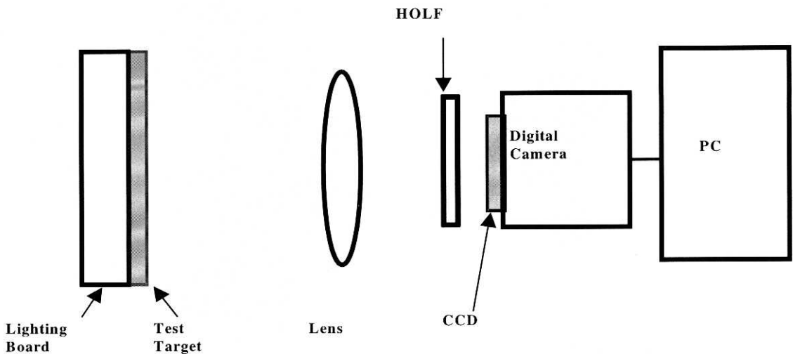
그림 5. HOLF 실장 실험을 위한 장치도.
