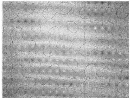
그림 4. 제작된 21 빔 HOLF의 현미경 사진. 홀로그래프의 주기는 280 \mu m이다.
