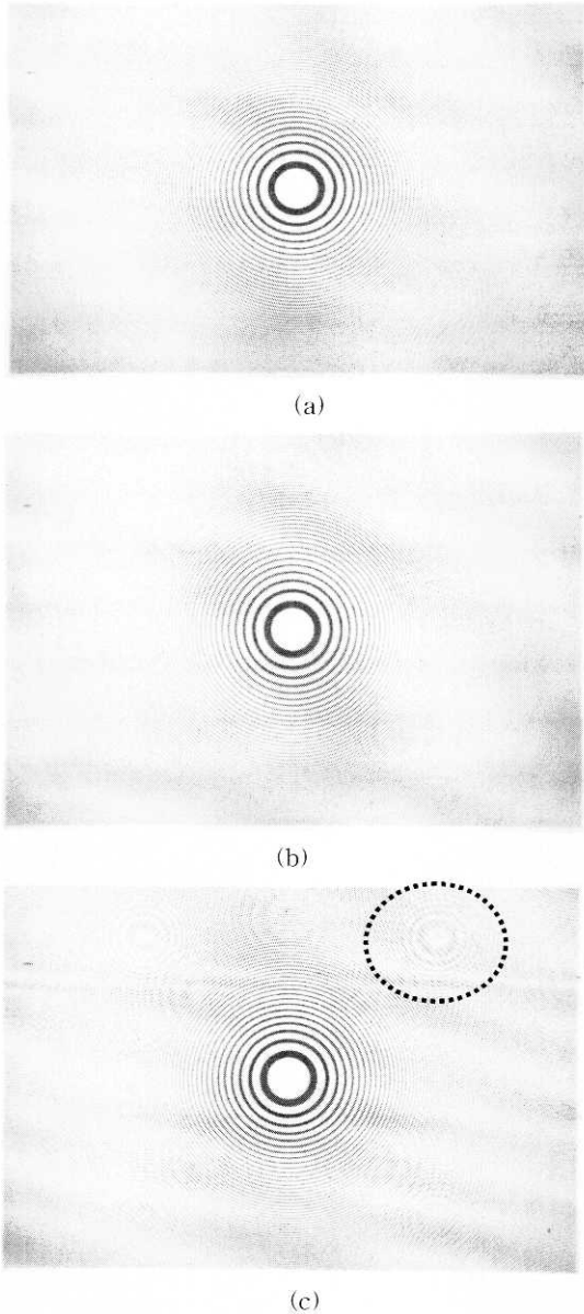
그림 6. 실장 실험용 카메라로 촬영한 zone plate의 상. (a) HOLF를 장착한 경우, (b) GOLF를 장착한 경우, (c) 광 저대역 필터가 없는 경우.
