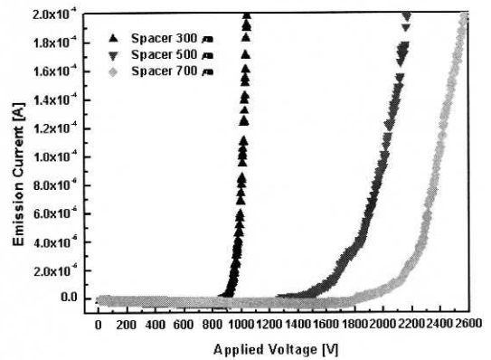
(a) spacer가 변화할 때의 방출전류
