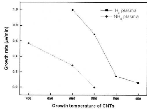
그림 6. NH 3 , H 2 gas plasma에서 탄소나노튜브 성장온도에 따른 성장률. Fig. 6. The growth rate of carbon nanotubes as a function of the growth temperature during NH 3 , H 2 gas plasma process.
