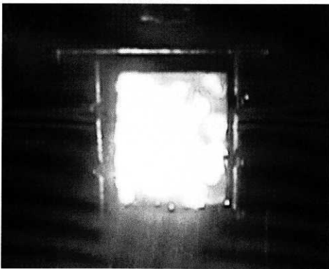
그림 10. 탄소나노튜브의 전계방출 모습. Fig. 10. Field emission image of CNTs.
