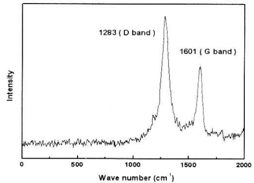
그림 7. 탄소나노튜브의 라만 스펙트라. Fig. 7. Raman spectra of the CNTs.
