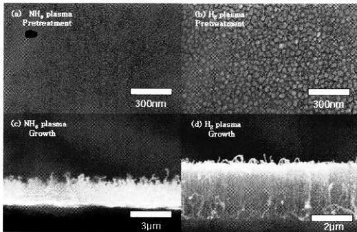
그림 4. NH 3 , H 2 gas에 따른 전처리 및 탄소나노튜브 성장. Fig. 4. Pretreatment & growth of the CNTs by NH 3 , H 2 gas.
