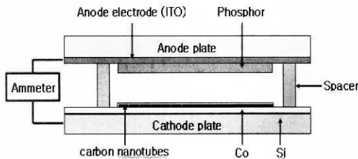
그림 2. 탄소나노튜브의 진계방출 특성을 측정하기 위한 평판 이극관 램프의 기하학적 구조.
