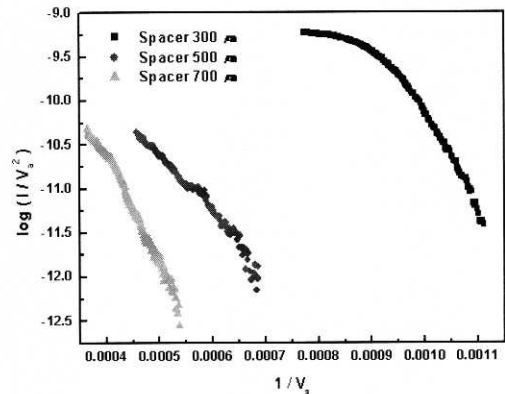
(b) 방출전류의 Fowler-Nordheim Plot
