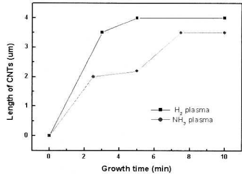
그림 5. 탄소나노튜브의 성장 시간 Vs 성장 길이. Fig. 5. Growth time Vs length of the CNTs.
