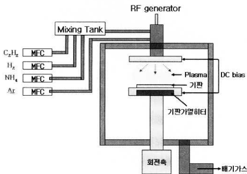
그림 1. PECVD 장비의 개략도.
