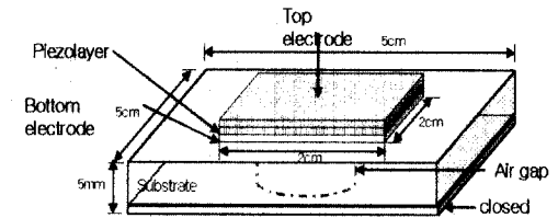
(b) 밀폐형
