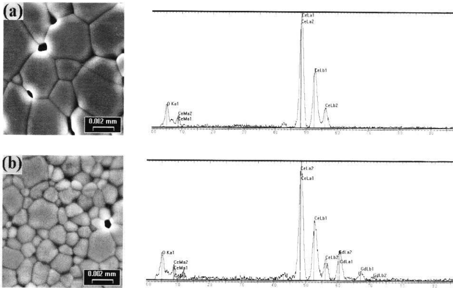
그림 5. (a) CeO_2 와 (b) 10 mol% Gd_2O_3 -doped CeO_2 의 SEM 사진과 EDX 스펙트럼.
