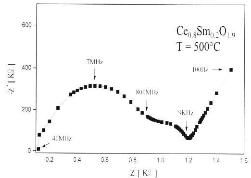
그림 6. Ce_{0.8}Sm_{0.2}O_{1.9} 세라믹스의 복소임피던스 다이어그램.
