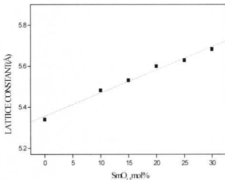
그림 4. Sm_2O_3 함량에 따른 CeO_2 의 격자상수 변화. Fig. 4. Lattice constant as a function of Sm_2O_3 content.
