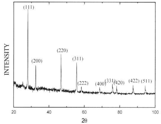
그림 1. Ce_{0.8}Sm_{0.2}O_{1.9} 세라믹스의 XRD패턴.
