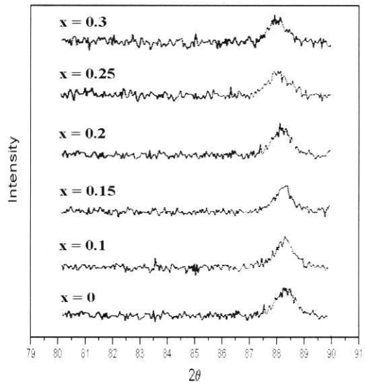
그림 2. Ce_{1-x}Gd_xO_{2-x/2} 세라믹스의 고각도 XRD패턴.
