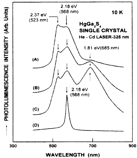
그림 3. HgGa 2 S 4 단결정의 광발광 특성.
