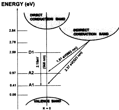
그림 7. HgGa 2 S 4 (A) 단결정의 Energy Band 모형. Fig. 7. Energy band diagram of HgGa 2 S 4 (A) single crystal.
