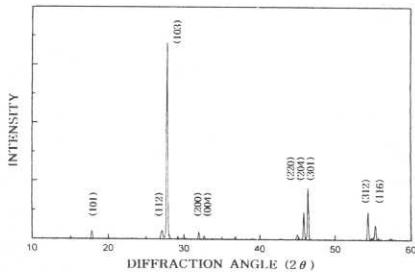
그림 3. CuAlSe 2 다결정의 X-선 회절 무늬. Fig. 3. X-ray diffraction patterns of CuAlSe 2 polycrystal.
