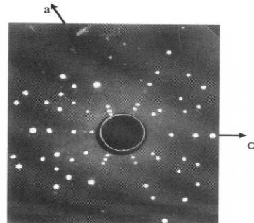
그림 6. 배면 반사법으로 측정된 (112)면의 Laue 무늬. Fig. 6. Back-reflection Laue patterns for the (112) plane.
