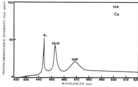
그림 12. Cu 분위기에서 열처리된 CuAlSe 2 단결정 박막의 10 K에서 PL 스펙트럼.
