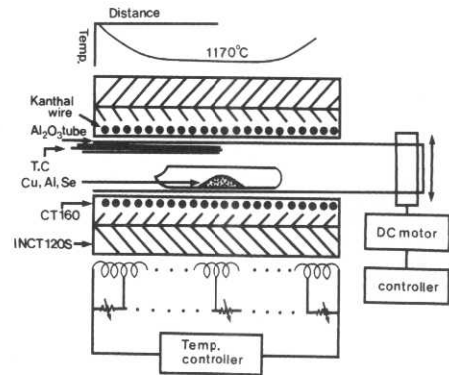
그림 1. \text{CuAlSe}_2 다결정 합성 수평 전기로.
