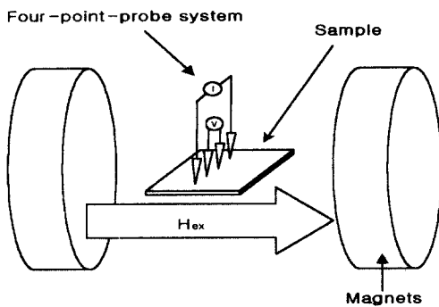
그림 1. 이방성자기저항비 측정장치의 개략도.
