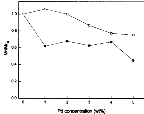
그림 4. Pd 조성 변화에 따른 정규화된 각형비의 변화.
