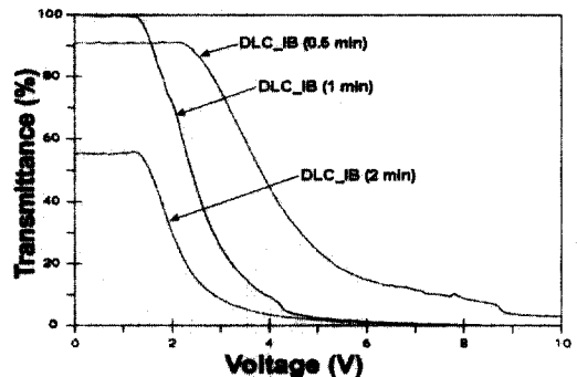
그림 3. DLC 박막 표면을 이용한 ion beam 배향 TN-LCD의 V-T 곡선.
