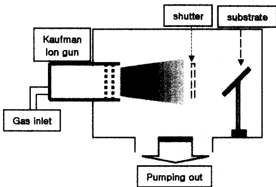
그림 1. Ion beam 조사 시스템.
