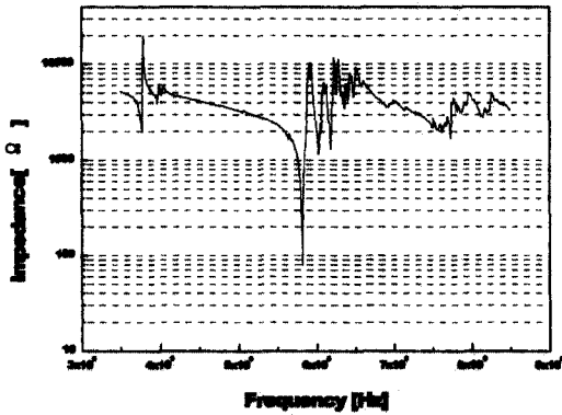
(b1) 전극직경 1.13mm 기본모드
