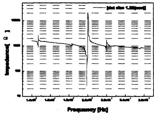
(c2) 전극직경 1.25mm 3차모드
