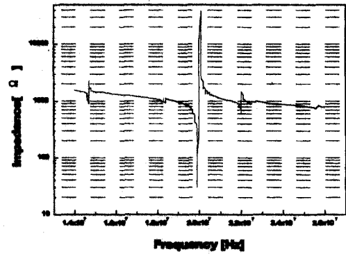
(b2) 전극직경 1.13mm 3차모드
