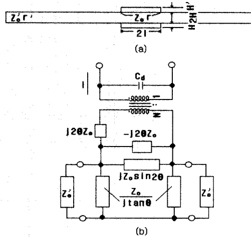
그림 1. 압전공진자와 분포정수등가회로.
