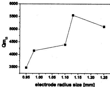
그림 3. 전극직경크기에 따른 Q_{m3} 의 변화.
