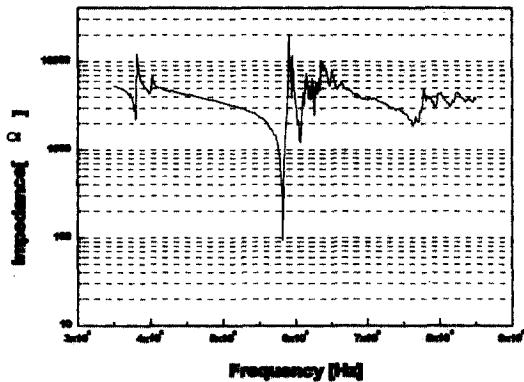
(c1) 전극직경 1.25mm 1차모드
