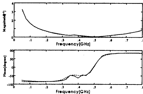
그림 7. 테스트 구조 2에 대한 측정된 Y11과 최적화된 Y11의 비교.
