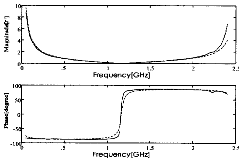
그림 6. 테스트 구조 1에 대한 측정된 Y11과 최적화된 Y11의 비교.
