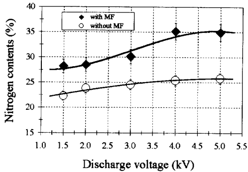
그림 2. 0.1 Torr에서 증착한 시료들의 방전 전압(kV)에 따른 질소 함유량 변화.
