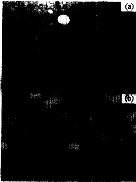
그림 5. 자장의 도움 무(a)와 도움 유(b) 일 때 증착한 시료의 SEM 이미지. 흰색 바는 1 \mu m 크기 임.
