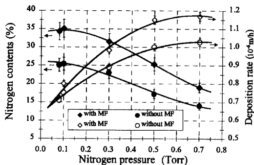
그림 3. 방전전압 4.0 kV에서 증착한 시료의 질소 압력에 따른 질소함유량과 증착속도.
