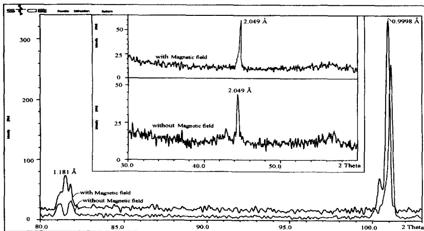
그림 6. 자장의 도움이 없을 경우와 도움을 가지고 증착된 시료의 XRD 스펙트럼 패턴.
