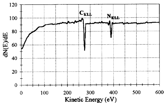
그림 1. 자장의 도움이 없이 0.1 Torr, 4.0 kV에서 증착한 두께가 1.4 \mu\text{m} 인 질화탄소 시료의 Auger 전자 스펙트럼.
