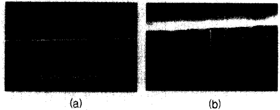
그림 6. 매몰 cavity를 갖는 SDB SOI 구조의 (a) 횡단면 및 (b) 확대 SEM 사진.
