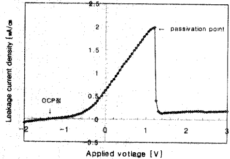
그림 3. P형 Si 기판의 누설전류-전압 특성곡선.
