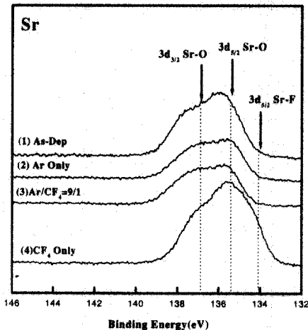
그림 4. CF 4 /(CF 4 +Ar) 가스 혼합비에 따라 식각된 BST박막 표면의 Sr 3d XPS narrow scan 스펙트럼.
