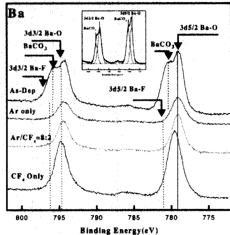
그림 3. CF 4 /(CF 4 +Ar) 가스 혼합비에 따라 식각된 BST박막 표면의 Ba 3d XPS narrow scan 스펙트럼.
