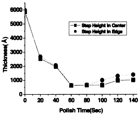
그림 6. 연마 시간에 따른 넓은 필드 산화막 지역에서 단차.
