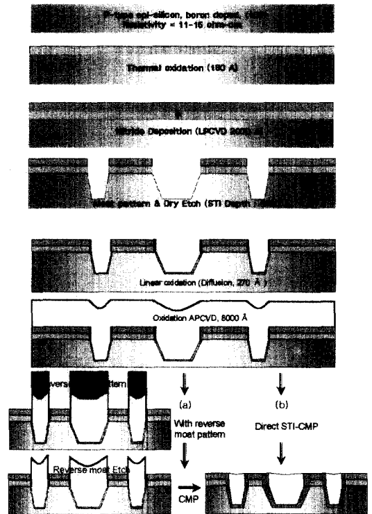
그림 1. STI 패턴 웨이퍼의 제조 순서도.
