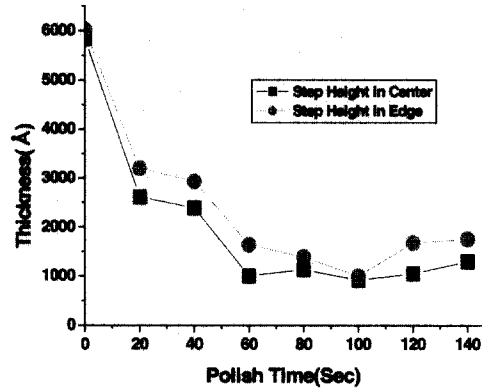
그림 7. 연마 시간에 따른 좁은 필드 산화막 지역에서 단차
