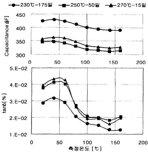
그림 12 복합가속열화 샘플에 대한 정전용량과 유전손실의 온도의존성.
