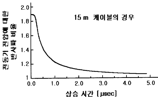
그림 3 상승시간에 대한 반사파 비율.
