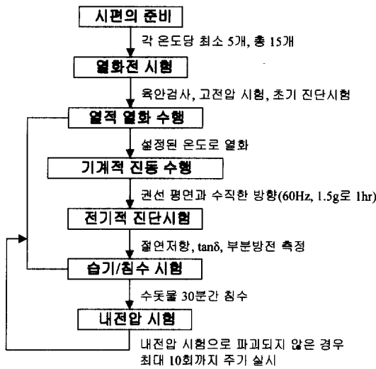
그림 5. C종 절연시스템의 복합가속열화 절차.
