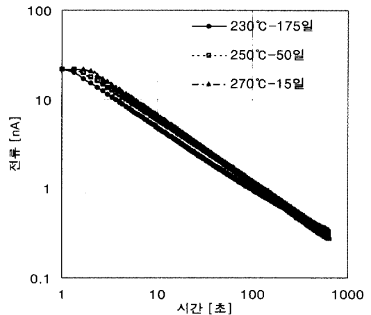
그림 6. 이중로그 척도의 분극전류 시간의존성(직류 1000V 인가, 40℃ 측정).
