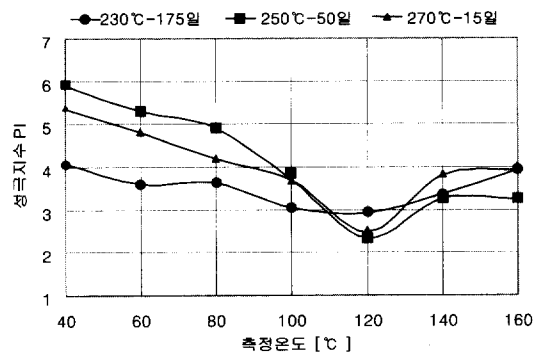
그림 8. 성극지수(PI) 특성의 온도 의존성. Fig. 8. Temperature dependency of polarization index(PI).
