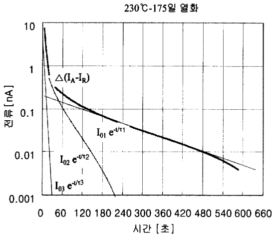
그림 10. 분극전류 \Delta(I_A - I_R) 의 성분분리를 위한 세미로그척도(230℃-175일 열화샘플, 40℃ 측정).
