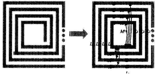
그림 4. 인덕턴스 계산을 위해 단순화된 spiral line의 구조.
