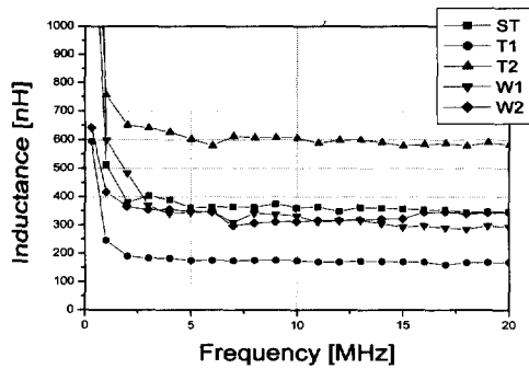
(a) 인덕턴스
