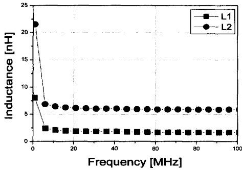
(a) 인덕턴스
