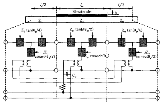
그림 5. Smith 등가회로모델. Fig. 5. Smith Equivalent circuit model.
