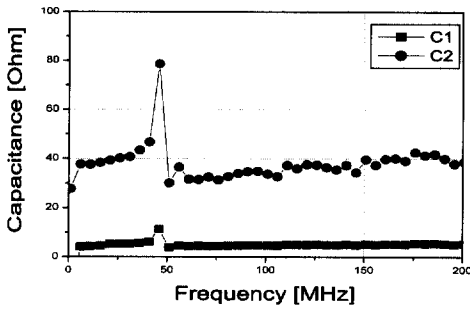
그림 9. Interdigital 형 커패시터의 측정결과. Fig. 9. Experimental result with interdigital type capacitors.
