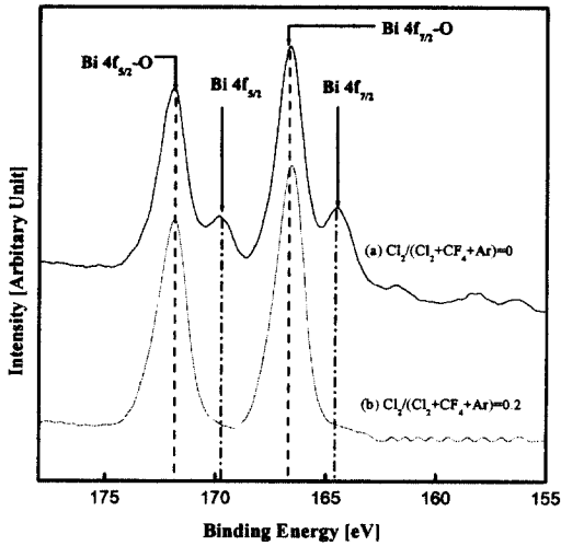
그림 3. Cl 2 가스 혼합비에 따라 식각 된 SBT 박막 표면에서 추출한 Bi 4f XPS narrow scan 스펙트럼. (a) Cl 2 /(Cl 2 +CF 4 +Ar)=0 (b) Cl 2 /(Cl 2 +CF 4 +Ar)=0.2
