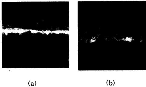
그림 7. 식각 후 SEM을 이용하여 촬영한 SBT 박막의 식각 단면 사진.(a) Cl_2/(Cl_2+CF_4+Ar)=0 , (b) Cl_2/(Cl_2+CF_4+Ar)=0.2
