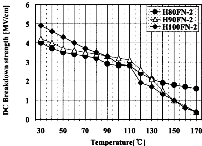
그림 2. 경화제 첨가 비율에 따른 직류 절연 파괴 강도. Fig. 2. DC breakdown strength according to ratio of adding hardener.
