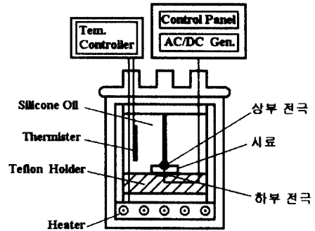
그림 1. 실험장치. Fig. 1. Experimental apparatus.
