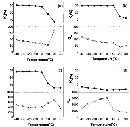
그림 4. 0.9PMN-0.1PT + x wt% MnO 2 에서 온도 변화에 따른 K_p 및 Q_m 의 변화. x=0 (a), x=0.1 (b), x=0.5 (c), x=1 (d).
