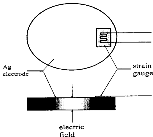
그림 1. 스트레인 측정을 위한 시편의 형상. Fig. 1. Shape of samples for strain measurement.
