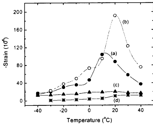
그림 5. 0.9PMN-0.1PT + x wt% MnO 2 에서 온도 변화에 따른 전계유기 변형 거동. x=0 (a), x=0.1 (b), x=0.5 (c), x=1 (d).
