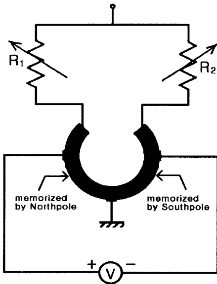
그림 9. 휘스톤 브리지형 자기 · 자극 센서. Fig. 9. Wheatstone bridge including magnetic field · polarity sensor.
