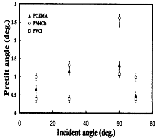
그림 2. 3종류의 광폴리머 표면에 편광된 UV 광을 1분간 조사시의 입사각도에 따른 프리틸트각의 발생.
