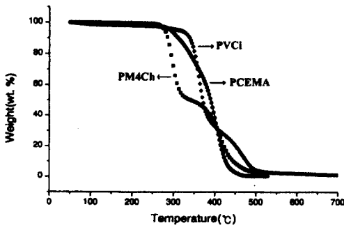
그림 4. 3종류의 광폴리머의 TGA 특성. Fig. 4. TGA characteristics of the three kinds of photo-polymer.
