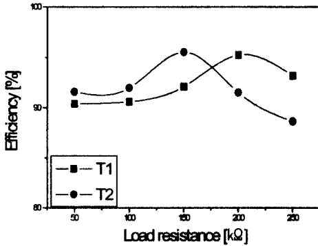
그림 6. 출력전력 6 W로 고정한 상태에서의 부하저항에 따른 효율. Fig. 6. Efficiency with load resistance under the fixed output power of 6 W.
