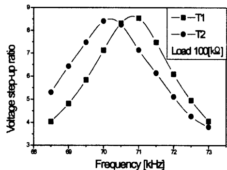
그림 8. 출력전력 6 W로 고정한 상태에서의 부하저항 100 kΩ에서의 주파수에 따른 승압특성. Fig. 8. Voltage step-up ratio as a function of frequency at load resistance 100 kΩ under the fixed output power of 6 W.
