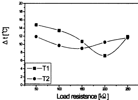
그림 7. 출력전력 6 W로 고정한 상태에서의 부하저항에 따른 온도상승. Fig. 7. Temperature rise with load resistance under the fixed output power of 6 W.
