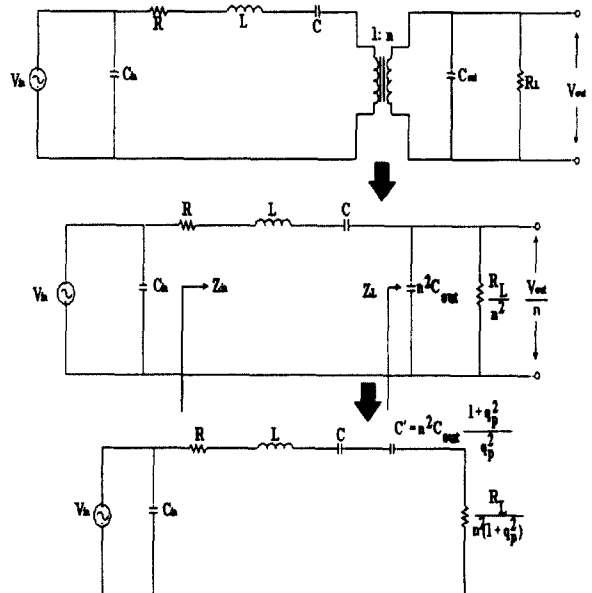
그림 1. 압전트랜스포머의 등가회로.
