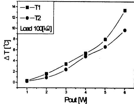
그림 10. 부하저항 100 kΩ에서의 출력전력에 따른 온도상승.
