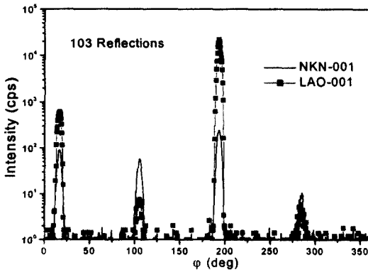
그림 5. Na 0.5 K 0.5 NbO 3 박막에서의 NKN과 LAO (103)-면에 대한 XRD ω 스캔
