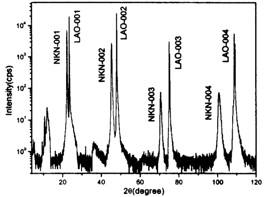
그림 3. Na 0.5 K 0.5 NbO 3 박막의 X선 회절 모양.
