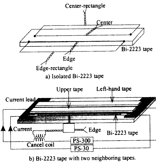
그림 1. 시료의 개략도.
