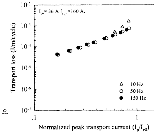
그림 6. 좌측테이프의 각 주파수에 대한 통전손실 - 정규화된 피크통전전류(가장자리 전압리드를 사용).
