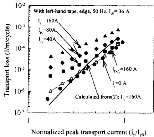
그림 5. 좌측 테이프의 각종 교류 전류에 대한 통전 손실 - 정규화된 피크 통전전류(가장자리 전압리드를 사용).
