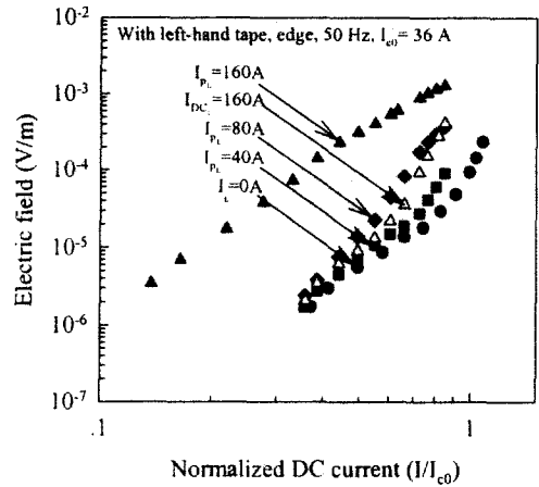
그림 4. 좌측테이프의 각종 교류전류에 대한 전계 - 정규화된 직류 통전전류(가장자리 전압리드를 사용).
