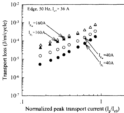
그림 7. 인접 테이프의 각종 배치방법에 대한 통전손실 - 정규화된 피크 통전 전류(가장자리 전압리드를 사용).
