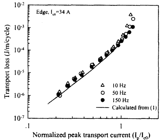
그림 3. 통전전류의 각종 주파수에 대한 통전손실 - 정규화된 피크 전류(가장자리 전압리드 사용).
