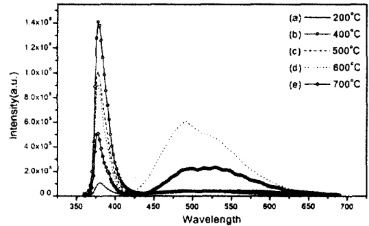
그림 1. 산소압 350 mTorr, 기관온도 (a) 200°C, (b) 400°C, (c) 500°C, (d) 600°C, (e) 700°C에서 (001) 사파이어 기관 위에 증착시킨 ZnO 박막의 PL 특성.
