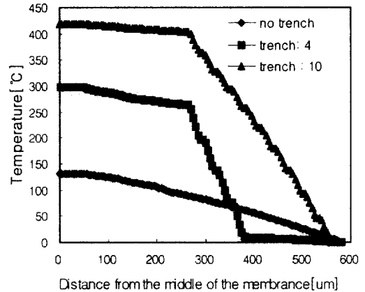
그림 3. SOI 멤브레인위의 트랜치 갯수와 멤브레인의 중앙에서부터 거리에 따른 미세발열체의 FDM 시뮬레이션 온도 분포도.
