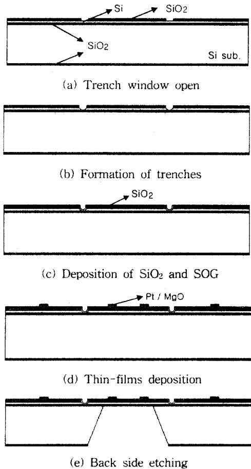
그림 1. SOI 멤브레인상에 트렌치를 갖는 미세발열체의 제작공정 순서도.
