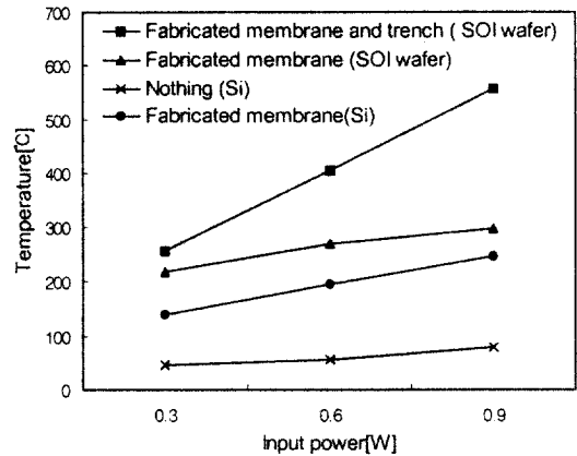
그림 8. 실리콘, 실리콘 멤브레인 그리고 트랜치를 갖는 SOI 멤브레인위에 각각 제조된 미세발열체의 발열특성.
