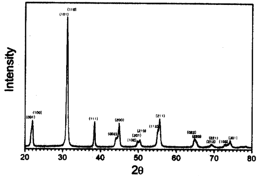
그림 3. 200°C에서 2시간 소결된 Pb[(Mn_{1/3}Sb_{2/3})_{0.05}Zr_{0.475}Ti_{0.475}]O_3 세라믹스의 X-선 회절분석.
