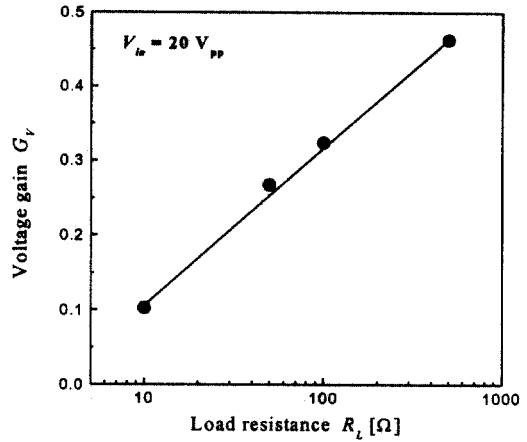
그림 7. 입력전압이 20 V pp 인 경우 전압이득과 부하저항의 상관관계.
