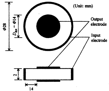
그림 1. 감압용 압전 트랜스포머의 모식도. Fig. 1. Schematic diagram of step-down piezoelectric transformer.
