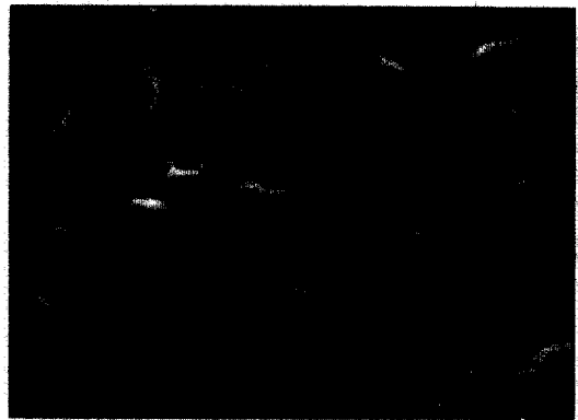
그림 4. 1200°C에서 2시간 소결된 Pb[(Mn_{1/3}Sb_{2/3})_{0.05}Zr_{0.475}Ti_{0.475}]O_3 세라믹스의 미세구조.
