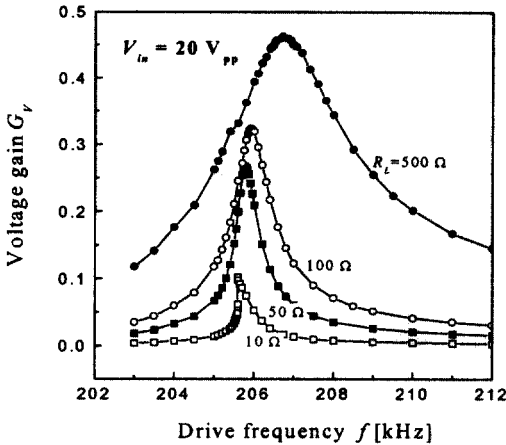
그림 6. 구동 주파수 및 부하저항에 따른 감압 트랜스포머의 전압이득.
