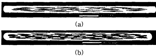
그림 1 Bi-2223/Ag 고온초전도 선재의 단면 형상 (a) 19심, (b) 37심
