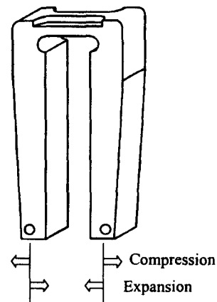
그림 2 Bi-2223/Ag 고온초전도 선재용 U-자형 치구
