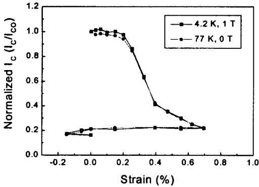
그림 5 다른 온도(77, 4.2 K) 및 자장(B=0, 1 T)하에서 측정된 변형을 대 임계전류
