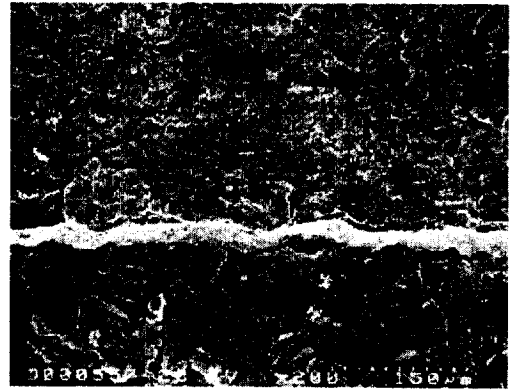
그림 6 19심 선재의 초전도 필라멘트간 균열 전파 Fig. 6 Fracture propagation between the superconducting filaments of 19 filamentary tapes.
