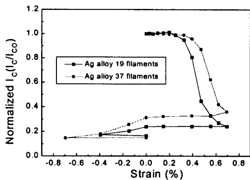
그림 4 변형-임계전류 측정에 따른 필라멘트 개수의 영향
