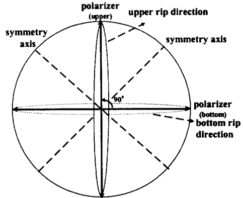
그림 4 수직 광폴리머를 이용한 새로운 MVA 셀 구조의 top view Fig. 4 Top view of schematic diagram of the new MVA cell using a homeotropic photopolymer
