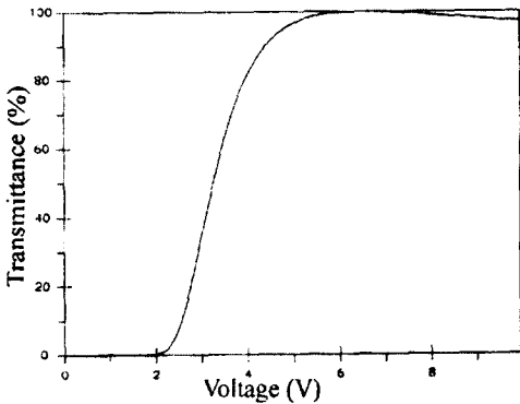
그림 6 러빙처리된 수직 폴리이미드 표면에서의 음의 보상 필름을 사용하지 않은 일반 VA 셀의 V-T 곡선
