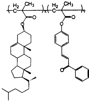
그림 1 광폴리머의 분자 구조 Fig. 1 Molecular structure of photopolymer
