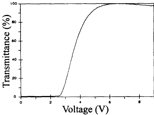
그림 5 수직 광폴리머를 사용한 새로운 MVA 셀의 전압-투과율 (V-T) 곡선
