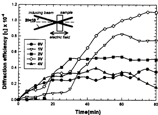
그림 3. As_{40}Ge_{10}Se_{15}S_{35} 박막의 수평 전압인가 변화에 의한 회절효율의 변화.
