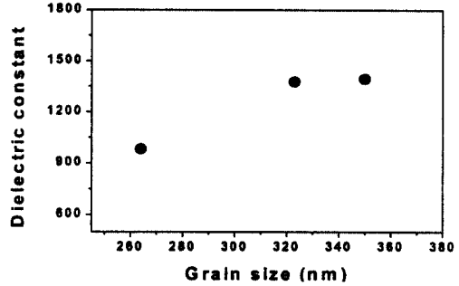
그림 4 그레인의 크기에 따른 PLT 박막의 유전상수 변화
