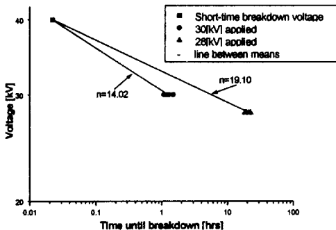
그림 7. 12500[cSt] 실리콘 오일을 도포한 시료의 V-t 특성
