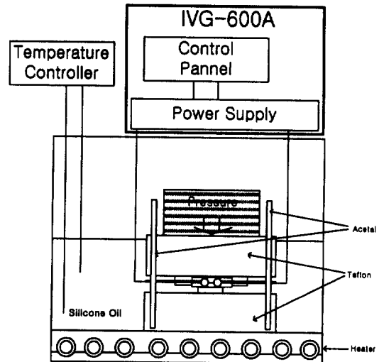
그림 2. 계면 절연내력 시험장치
