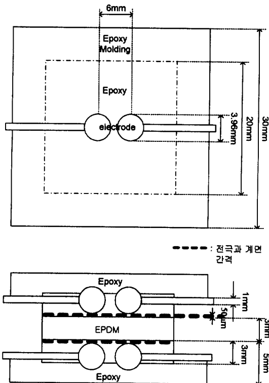
그림 1. 제작된 시료의 구조 Fig. 1. Structure of specimen
