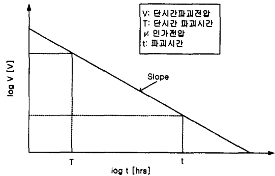
그림 4. V-t 특성도
