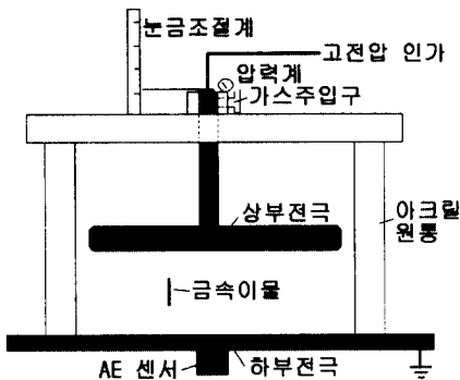
그림 2. 모의 GIS Fig. 2. Gas Insulated Switchgear
