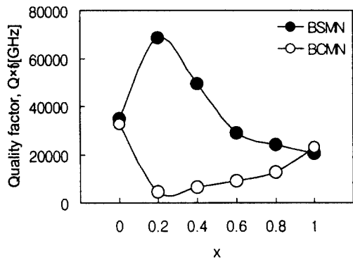
그림 8. BSMN과 BCMN계 세라믹스의 품질계수.
