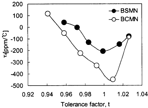
그림 7. BSMN 및 BCMN계의 관용계수에 대한 유전율의 온도계수.
