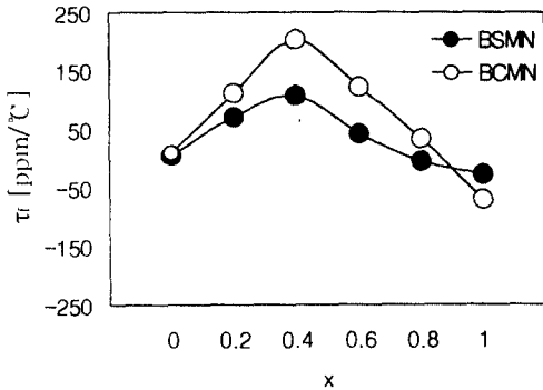
그림 9. BSMN과 BCMN계 세라믹스의 공진주파수의 온도계수. Fig. 9. Temperature coefficient of resonant frequency of BSMN and BCMN ceramics.
