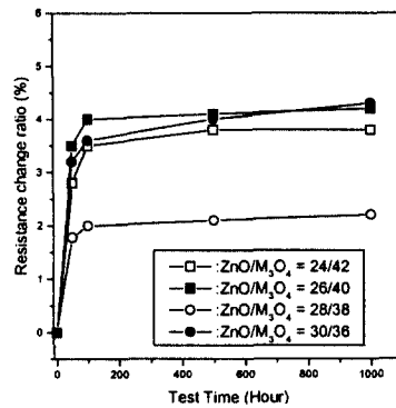
그림 7. ZnO/Mn 3 O 4 비에 따른 NTC 써미스터의 경시 변화
