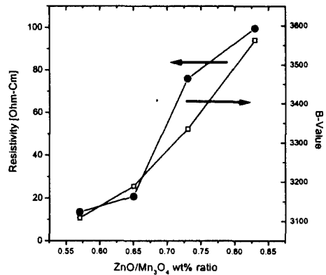
그림 2. ZnO/Mn 3 O 4 비에 따른 NTC 써미스터의 비저항 \rho_{25} 및 B-정수
