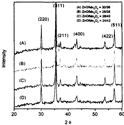
그림 1. ZnO/Mn 3 O 4 비에 따른 NTC 써미스터의 XRD 패턴
