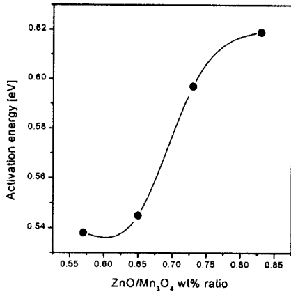
그림 3. ZnO/Mn 3 O 4 비에 따른 NTC 써미스터의 활성화 에너지
