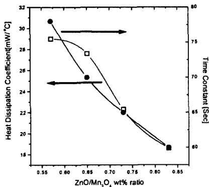
그림 6. ZnO/Mn 3 O 4 비에 따른 NTC 써미스터의 열방산정수 및 시정수
