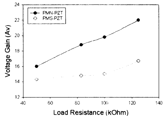
그림 12. 전압이득 특성 Fig. 12. Voltage set-up ratio characteristics
