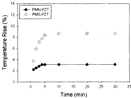
그림 13. 동작시간에 따른 온도상승 특성 Fig. 13. Temperature rise characteristics with variation of operating time
