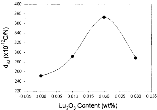
그림 6. PMS-PZT의 압전상수 Fig. 6. Piezoelectric constant of PMS-PZT
