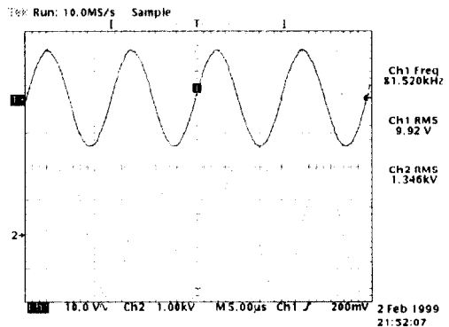
(a)PMS-PZT
