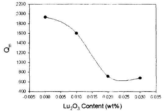
그림 8. PMS-PZT의 기계적 품질계수 Fig. 8. Mechanical quality factor of PMS-PZT
