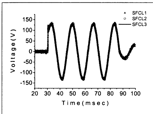
그림 3 개별 단위소자의 켄치 특성 (100 V rms ) Fig. 3 Quench characteristics of individual unit element (100 V rms )
