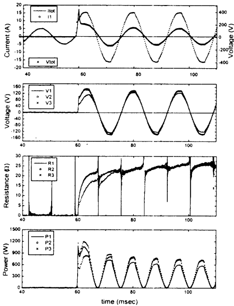
그림 5 SFCL1에 220 Ω 션트저항을 부착한 3개 단위 소자 직렬연결시 켄치 특성(300 V rms ) Fig. 5 Quench characteristics in serial connection of 3 SFCLs having a shunt resistor of 220 Ω into SFCL1 (300 V rms )
