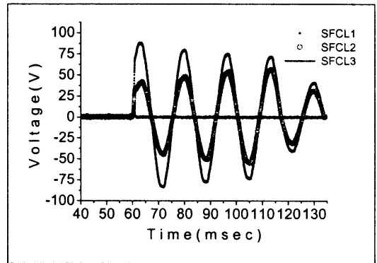
그림 4 단순 직렬연결시의 켄치특성 (100 V rms ) Fig. 4 Quench characteristics in simple serial connection (100 V rms )
