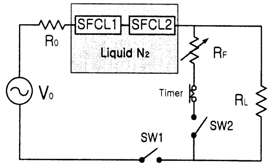
그림 2 실험회로도 (실험 목적에 따라 한류소자는 직·병렬 연결된다)
