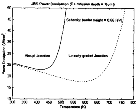
그림 3.13. 온도에 따른 접합장벽조절 쇼트키 정류기의 전력 소모.
