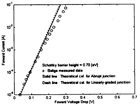
그림 3.6. 접합장벽조절 쇼트키 정류기의 순방향 전류-전압 특성 곡선.
