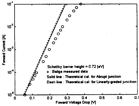
그림 3.5. 접합장벽조절 쇼트키 정류기의 순방향 전류-전압 특성 곡선.
