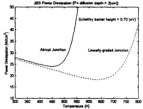
그림 3.14. 온도에 따른 접합장벽조절 쇼트키 정류기의 전력 소모.
