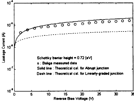
그림 3.9. 접합장벽조절 쇼트키 정류기의 역방향 전류-전압 특성 곡선. ( \phi_b=0.72 [eV], P+ 접합깊이=1[ \mu m]). Fig. 3.9. Reverse I-V characteristics of junction barrier controlled schottky rectifiers. ( \phi_b=0.72 [eV], P+ junction depth=1 [ \mu m]).
