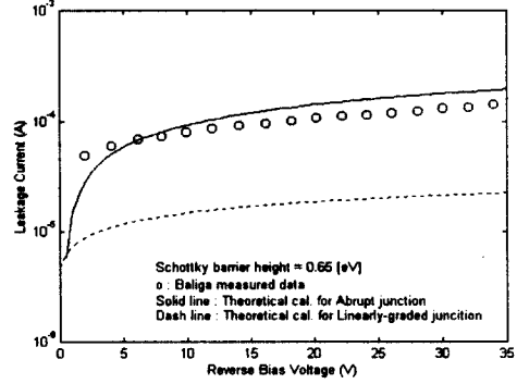
그림 3.11. 접합장벽조절 쇼트키 정류기의 역방향 전류-전압 특성 곡선. ( \phi_b=0.65 [eV], P+ 접합깊이=1[ \mu m]). Fig. 3.11. Reverse I-V characteristics of junction barrier controlled schottky rectifiers. ( \phi_b=0.65 [eV], P+ junction depth=1 [ \mu m]).
