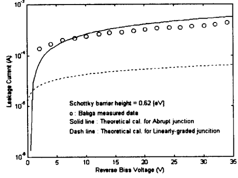
그림 3.12. 접합장벽조절 쇼트키 정류기의 역방향 전류-전압 특성 곡선. ( \phi_b=0.62 [eV], P+ 접합깊이=1[ \mu m]). Fig. 3.12. Reverse I-V characteristics of junction barrier controlled schottky rectifiers. ( \phi_b=0.62 [eV], P+ junction depth=1 [ \mu m]).
