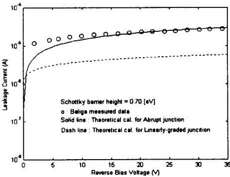
그림 3.10. 접합장벽조절 쇼트키 정류기의 역방향 전류-전압 특성 곡선. ( \phi_b=0.70 [eV], P+ 접합깊이=1[ \mu m]). Fig. 3.10. Reverse I-V characteristics of junction barrier controlled schottky rectifiers. ( \phi_b=0.70 [eV], P+ junction depth=1 [ \mu m]).
