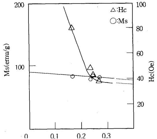
그림 6. Fe_{3-x}Ni_xO_4 막의 포화자화( M_s ) 및 보자력( H_c )의 조성 X 의존성
