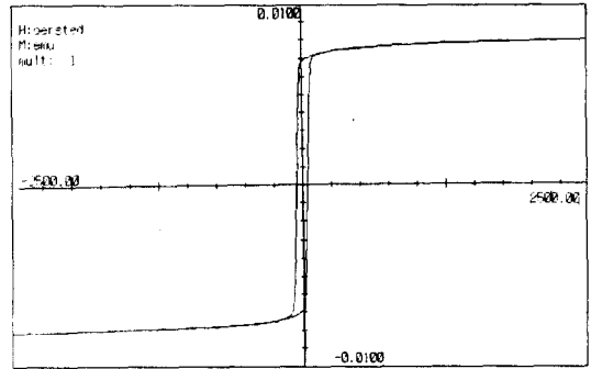
그림 5. S-85시편의 자기력곡선
