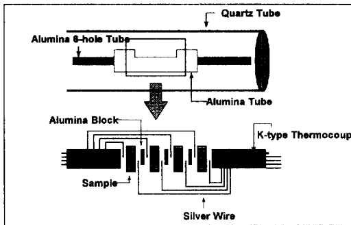
그림 1. 시편홀더 배치도.
