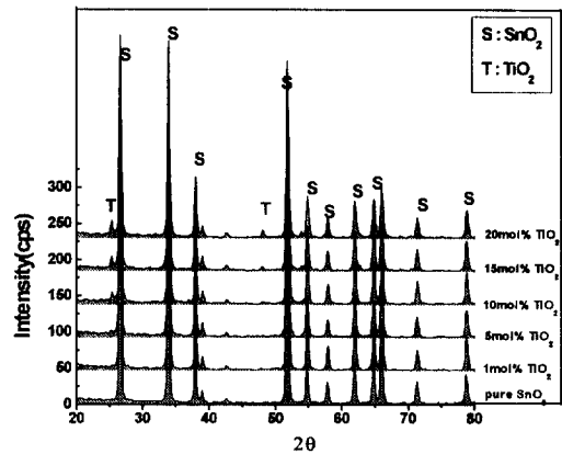
그림 2. TiO 2 첨가량에 따른 XRD 패턴.
