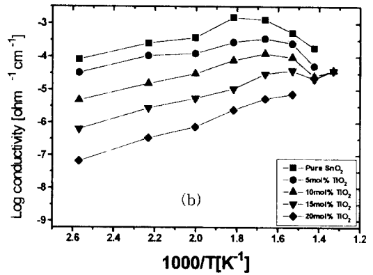
그림 4. 복합체 조성에 따른 전기전도도의 온도의존성.
