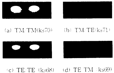
그림 6. 시편 도파모드 (P3), (OPELS, Tunable Semiconductor Laser, 1550 nm)
