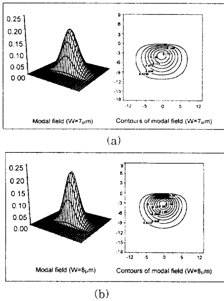
그림 8. 광전계 및 contour 분포(P2, TM mode) (a) 7\mu\text{m} 채널도파로 (b) 8\mu\text{m} 채널도파로 Fig. 8. Optical modal field and contour (a) 7\mu\text{m} 채널도파로 (b) 8\mu\text{m} 채널도파로
