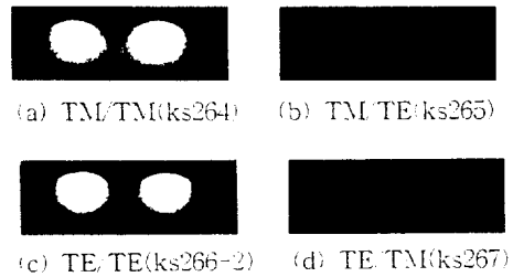
그림 5. 시편 도파모드(P2), (OPELS, Tunable Semiconductor Laser, 1550 nm)
