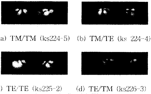
그림 10. 632.8nm HeNe laser 입사패턴 (p2) (a) TM/TM (b) TM/TE (c) TE/TE (d) TE/TM
