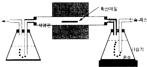
그림 1. 확산로 구조
