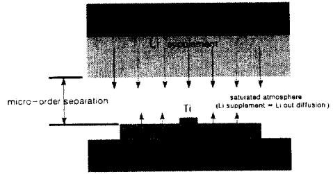
그림 2. Li 외확산 억제방법
