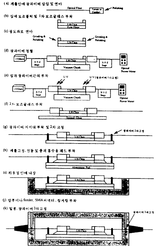
그림 12. 피그테일링 실험 Fig. 12. Experimental diagram of Pigtailing
