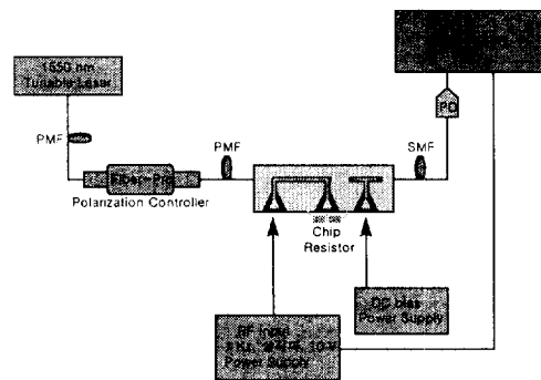
그림 13. 구동전압 측정 Fig. 13. Diagram of driving voltage measurement
