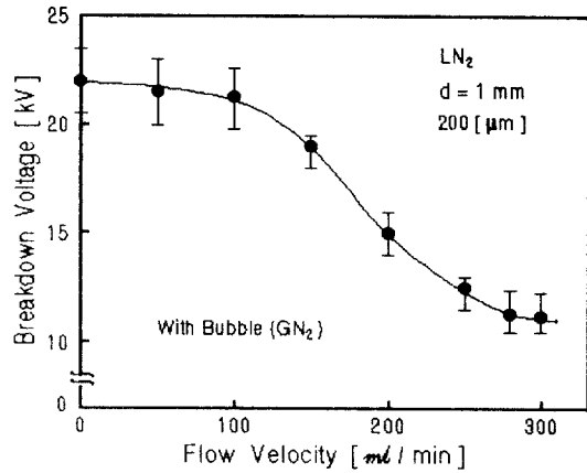
그림 7. 절연파괴전압에 미치는 유량의 의존성 Fig. 7. Dependence of flow capacity on breakdown voltage
