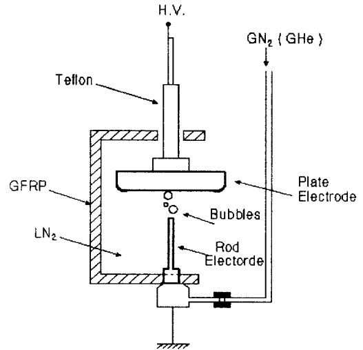
그림 2. 전극계 Fig. 2. Electrodes
