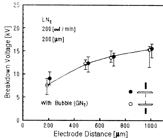
그림 8. LN 2 의 파괴전압의 전극배치 영향 Fig. 8. Dependence of electrode arrangements on breakdown voltage in LN 2
