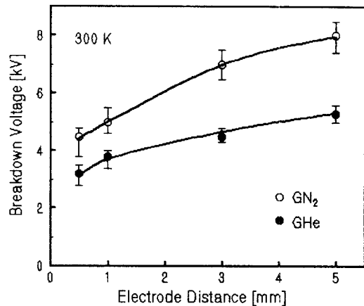
그림 5. GN 2 및 GHe의 절연파괴 특성 Fig. 5. Breakdown characteristic in GN 2 and GHe
