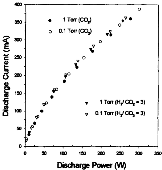
그림 5. 방전전력-전류특성
