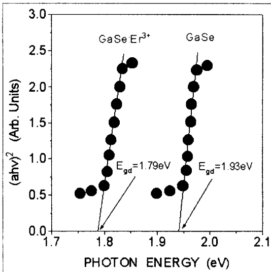
그림 4. GaSe와 GaSe:Er 3+ 단결정의 입사광 에너지 h\nu 대 (\alpha h\nu)^2 의 관계.
