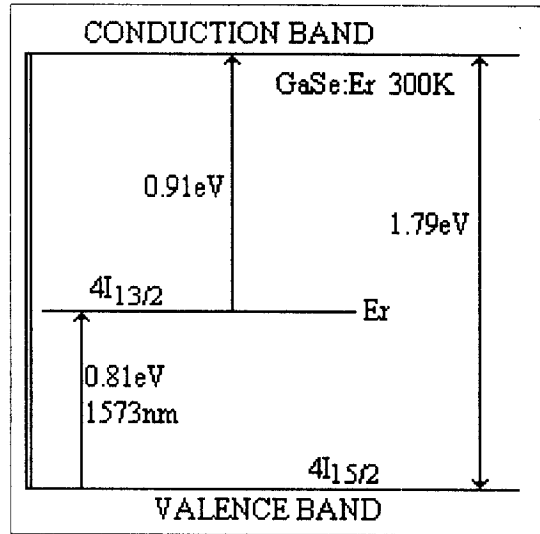
그림 7. GaSe:Er 3+ 단결정의 Er 3+ 에너지 준위.
