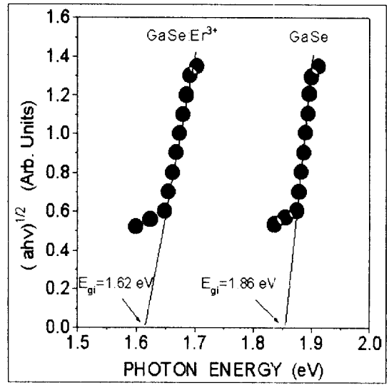
그림 5. GaSe와 GaSe:Er 3+ 단결정의 입사광 에너지 h\nu 대 (\alpha h\nu)^{1/2} 의 관계
