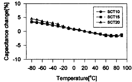
그림 3. 온도에 따른 정전용량의 변화 Fig. 3. Capacitance variation with temperature
