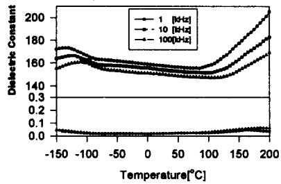
그림 5. 온도의 함수로서 유전상수와 유전손실의 주파수 의존성 Fig. 5. Frequency dependence of dielectric constant dielectric loss as a function of temperature
