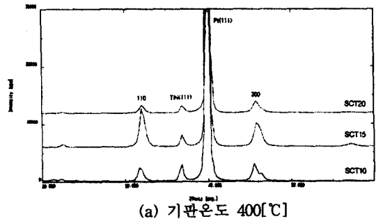
(a) 기판온도 400[°C]
