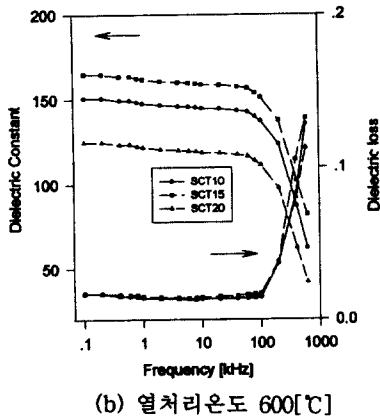
그림 4. 주파수에 따른 SCT 박막의 유전상수 및 유전 손실 Fig. 4. Dielectric constant and dielectric loss of SCT thin films with frequency
