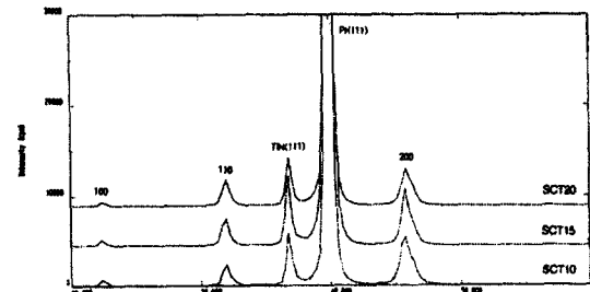
(b) 후속 열처리 600[°C]
