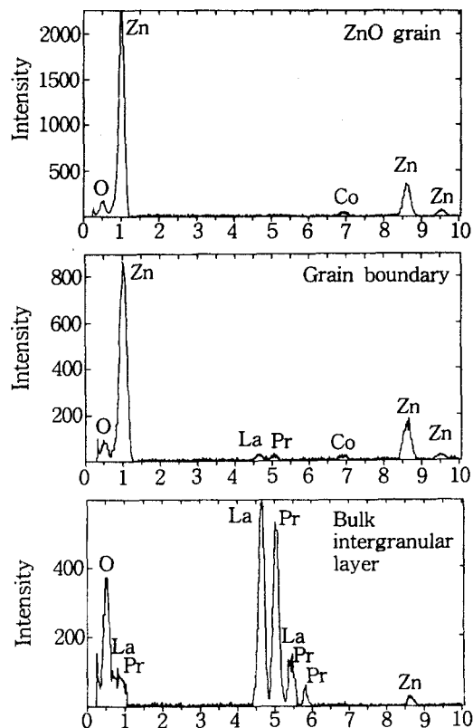
그림 2. 2.0mol% La 2 O 3 가 첨가된 Pr계 ZnO 바리스터 시편의 EDAX 패턴
