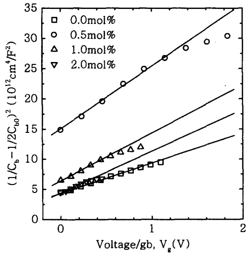
그림 7. \text{La}_2\text{O}_3 첨가량에 따른 Pr계 ZnO 바리스터의 변형된 C-V 특성
