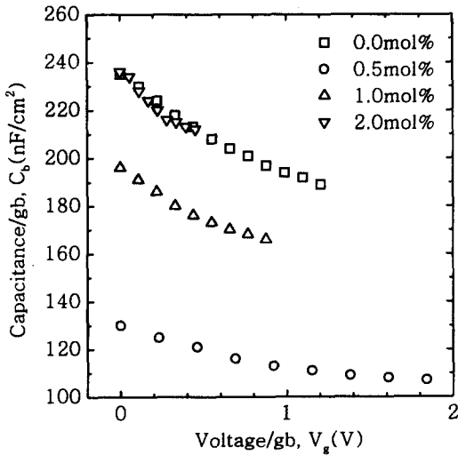
그림 6. \text{La}_2\text{O}_3 첨가량에 따른 Pr계 ZnO 바리스터의 C-V 특성
