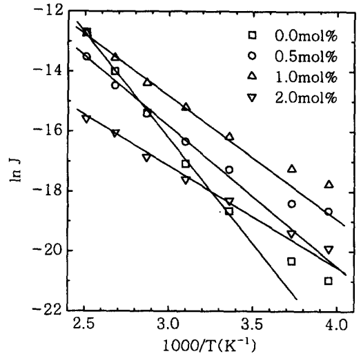
그림 4. La 2 O 3 첨가량에 따른 Pr계 ZnO 바리스터의 E=0에서 도시된 lnJ-1/T 특성
