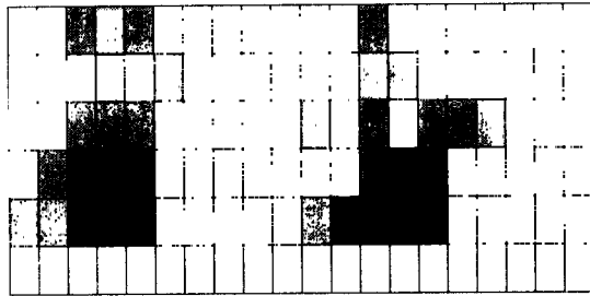
그림 12. 절연 상태의 파괴 직전 \phi -q-n 패턴 Fig. 12. \phi -q-n pattern at aging breakdown
