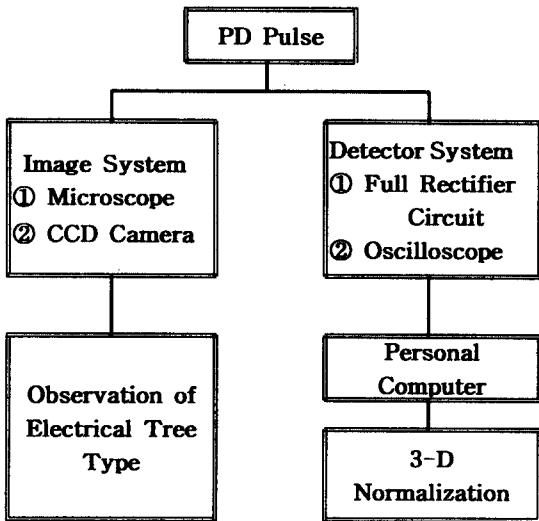
그림 3. 전기 트리 형상 및 방전 신호 검출 과정 Fig. 3. The acquiring process of discharge signal and electrical tree type
