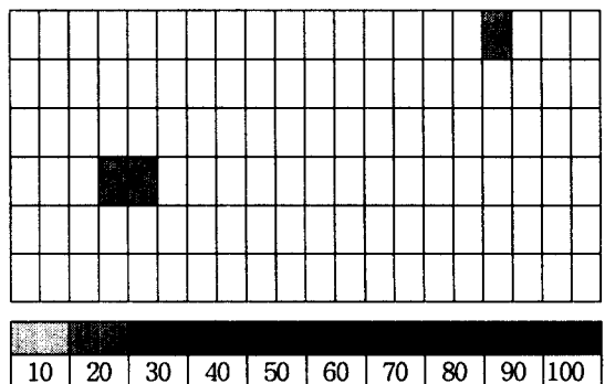
그림 10. 절연 열화 개시의 \varphi -q-n 패턴 Fig. 10. \varphi -q-n pattern on aging initiation
