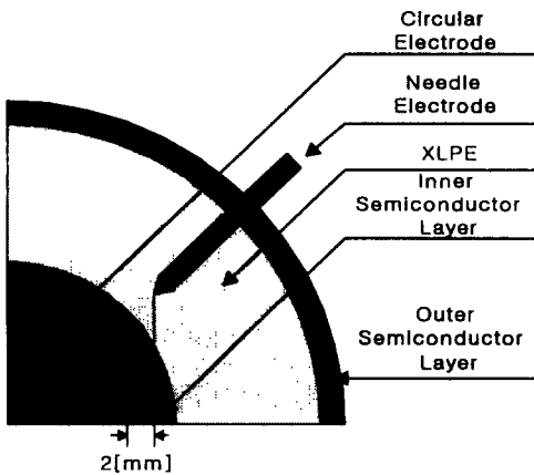
그림 1. 시료의 구조
