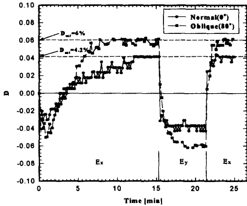
그림 5. 증착각도가 0°와 80°인 비정질 As 40 Ge 10 Se 15 S 35 박막에 선형 편광된 He-Ne 레이저 노출에 따른 광유기 이색성의 생성과 재방향.
