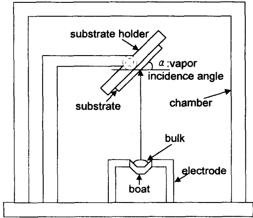
그림 2. 진공증착시스템. Fig. 2. Vacuum evaporation system.
