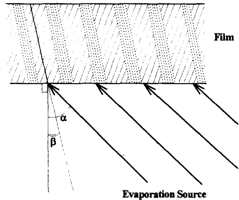
그림 4. 증착각도와 기둥각과의 관계. Fig. 4. The relation between deposition angle and columnar angle.
